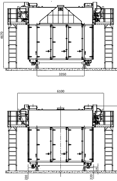
Desenho técnico: Modelo SHWZ/T 300x2
